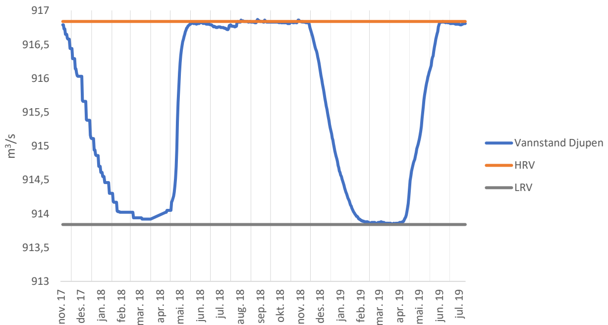
Figur 58. Magasin vannstand for Djupen i perioden november 2017 til juli 2019.
