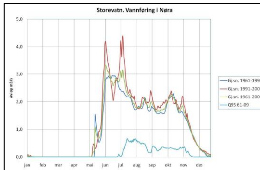
Figur 15: Avløp fra Storevatn til Nøra. Avløp eksklusive tapping gjennom reguleringsluke. Etterberegnet på grunnlag av oppmålinger i Nøra gjort av NVE høsten 2010, og magasin vannstander. Figur hentet fra bilag til FBRs revisjonsdokument for Åbjøravassdraget (2010).
