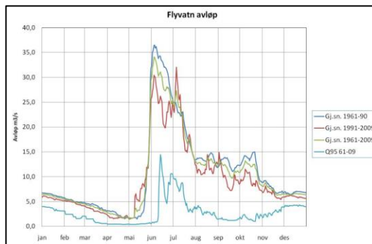
Figur 16: Avløp fra Flyvatn er summen av avløp over dam og gjennom luker. Etterberegnet på grunnlag av overløpskurve, vannstand i magasin og lukeåpninger. Figur hentet fra bilag til FBRs revisjonsdokument for Åbjøravassdraget (2010).
