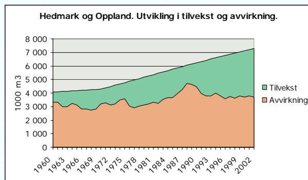
Figur 11: Fordi det stadig bygges opp mer og mer virke i norske skoger, bindes det også en større andel klimagasser i skog.
